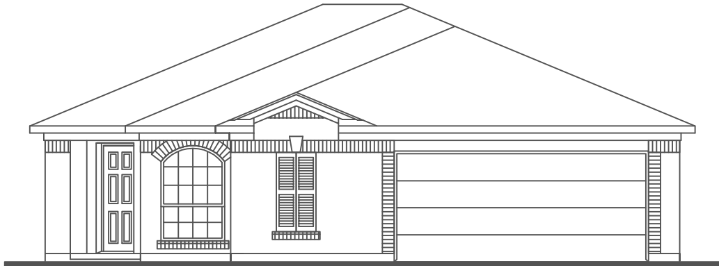
Elev "B"
